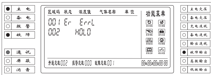
图-6 探测器连线故障
