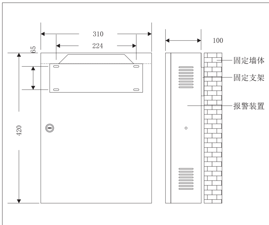
图-3 控制器的结构及安装尺寸
