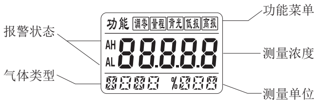
图-2 探测器的液晶
