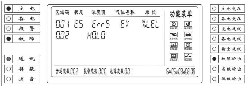
图-7 1号探测器传感器故障
