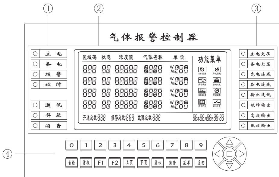
图-4 控制器面板
